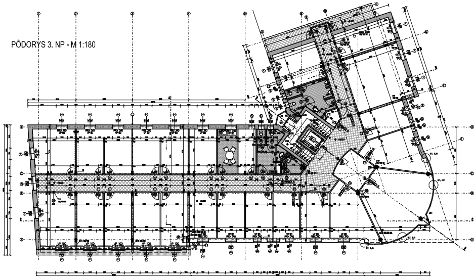
PÓDORYS 4. NP - M 1:180
