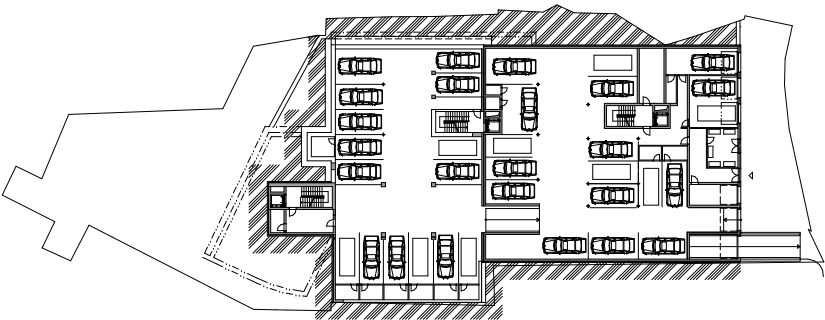
PÔDORYS 1. PP - M 1:400
