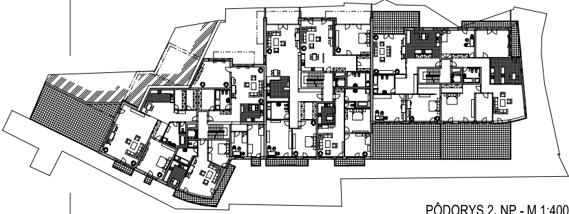
PÔDORYS 2. NP - M 1:400
