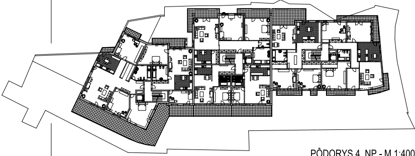
PÔDORYS 4. NP - M 1:400
