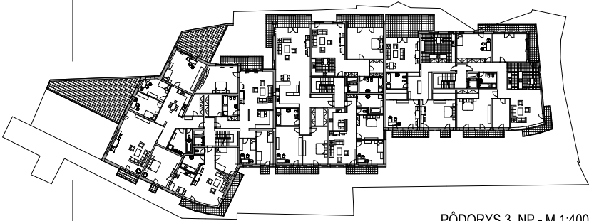
PÔDORYS 3. NP - M 1:400
