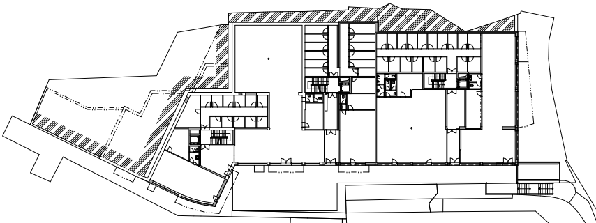
PÔDORYS 1. NP - M 1:400
