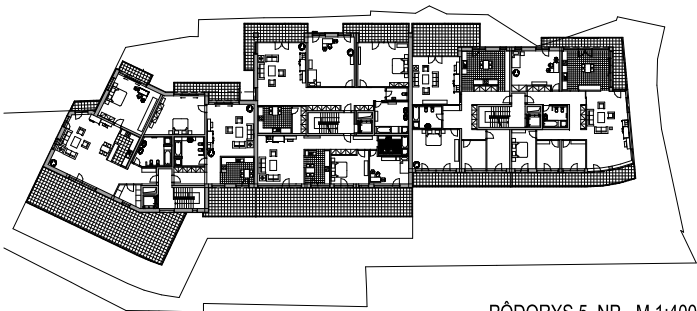
PÔDORYS 5. NP - M 1:400
