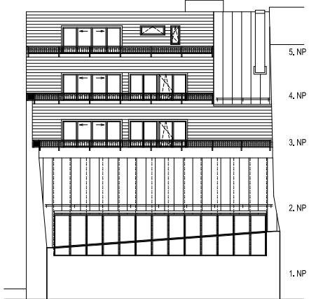
ZADNÝ POHĽAD - M 1:150
