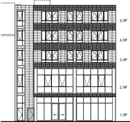
ČELNÝ POHĽAD - M 1:150
