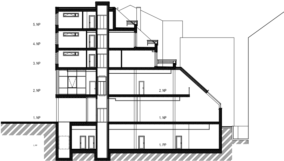
POZDĹŽNY REZ - M 1:150
