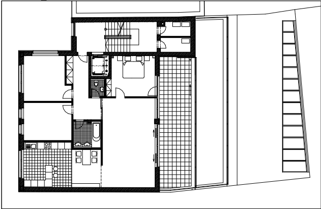
PÔDORYS 4.NP - M 1:150
