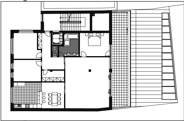
PÔDORYS 3.NP - M 1:150
