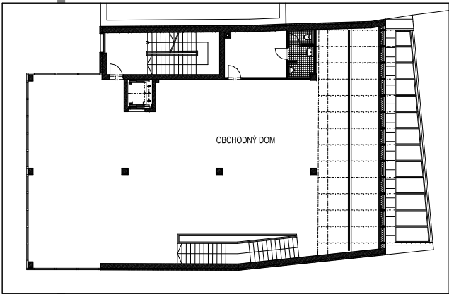
PÔDORYS 2.NP - M 1:150
