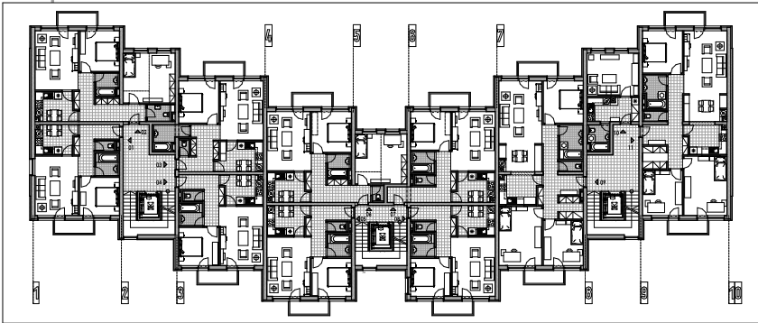
PÔDORYS 2. - 4. NP - M 1:250
