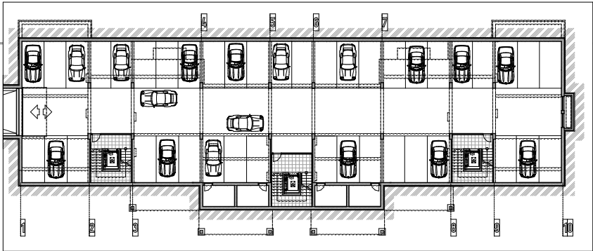
PÔDORYS 1. PP - M 1:250
