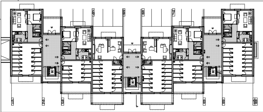
PÔDORYS 1. NP - M 1:250
