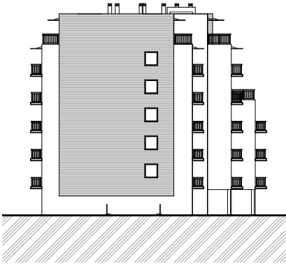
BOČNÝ POHĽAD - M 1:250
