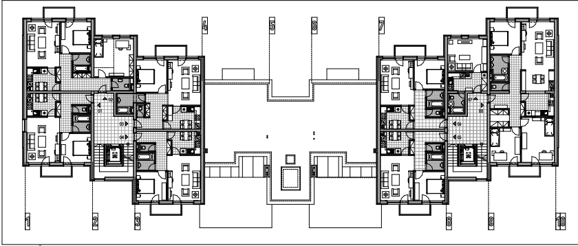
PÔDORYS 6. NP - M 1:250
