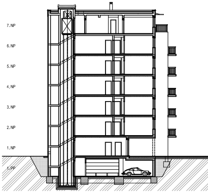
PRIEČNY REZ - M 1:250
