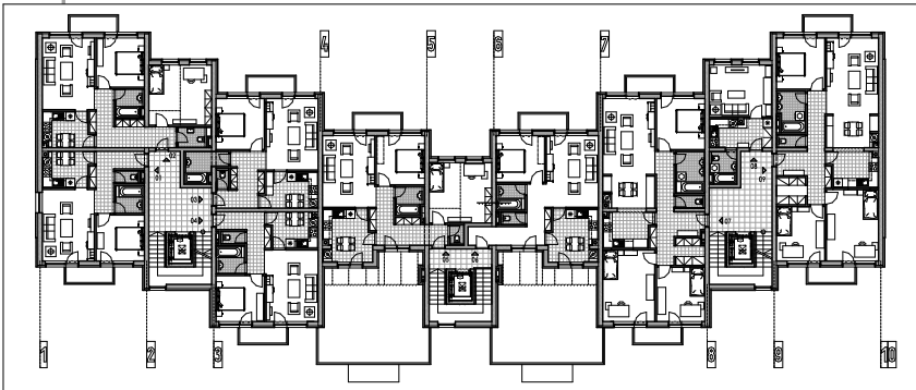
PÔDORYS 5. NP - M 1:250
