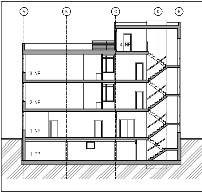
PRIEČNY REZ - M 1:200
