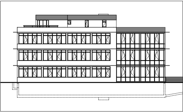
POHLAD BOČNÝ ĽAVÝ - M 1:200
