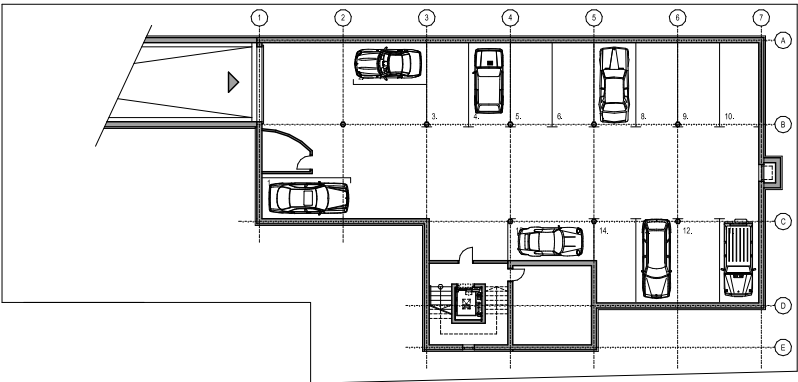
PÔDORYS 1. PP - M 1:200
