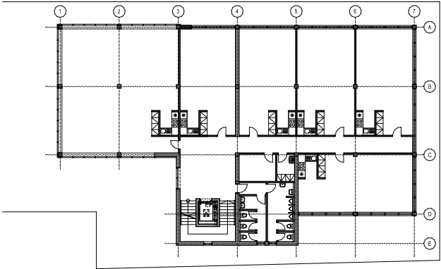
PÔDORYS 4. NP - M 1:200
