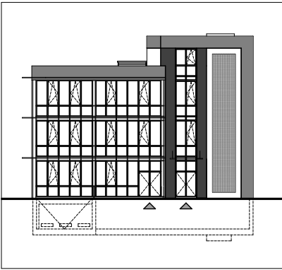
POHLAD ČELNÝ - M 1:200
