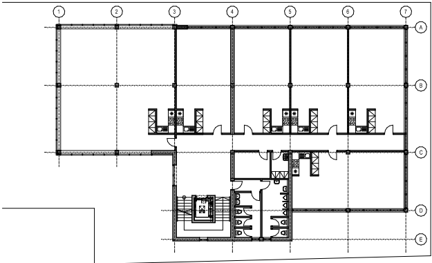
PÔDORYS 3. NP - M 1:200
