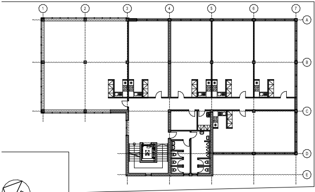
PÔDORYS 2. NP - M 1:200
