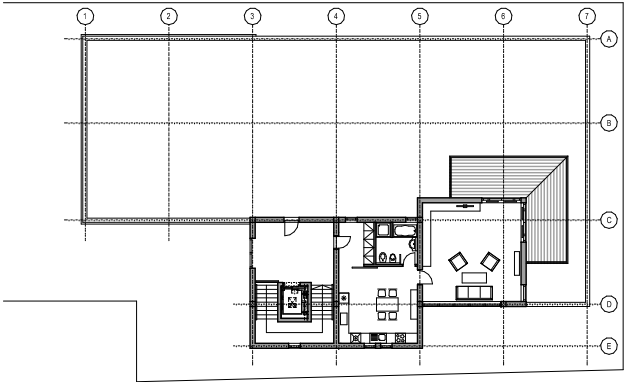
PÔDORYS 5. NP - M 1:200
