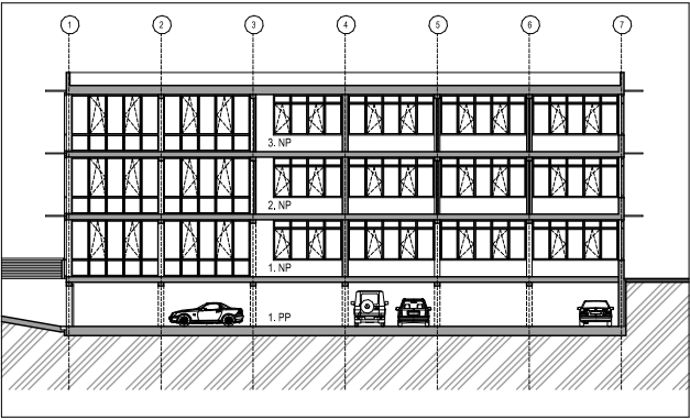
POZDĽŽNY REZ - M 1:200
