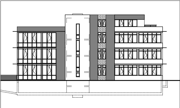
POHLAD BOČNÝ PRAVÝ - M 1:200
