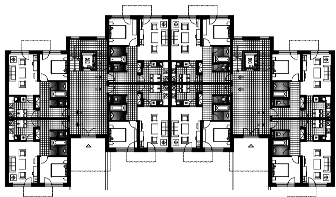
PŮDORYS 1. NP - M 1:200 BLOK B
