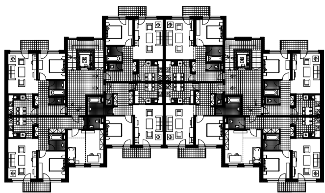
PŮDORYS 2. - 4. NP - M 1:200 BLOK B
