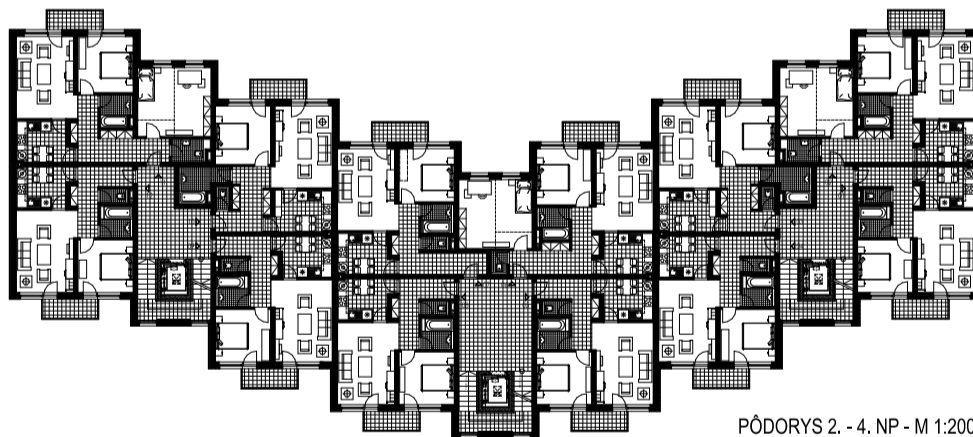
PŮDORYS 2. - 4. NP - M 1:200 BLOK A
