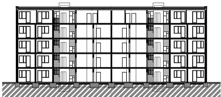
POZDĹŽNY REZ - M 1:200 BLOK B
