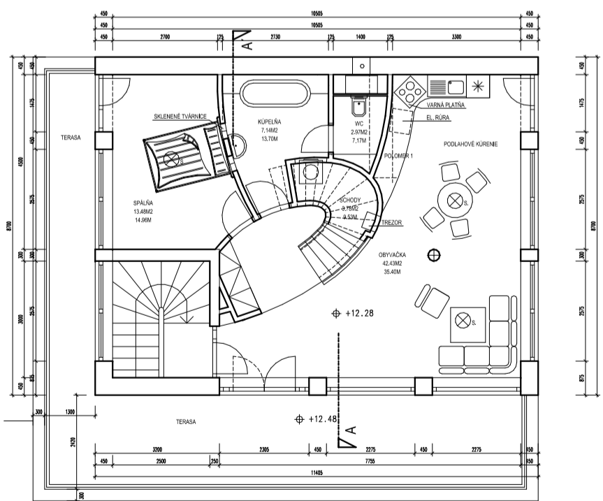
PÔDORYS 5. NP
