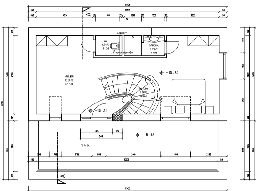
PÔDORYS 6. NP
