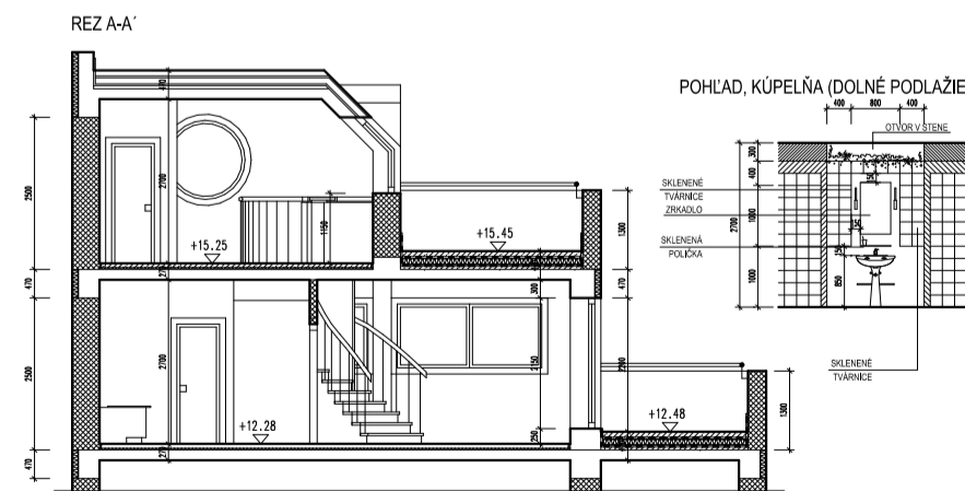
REZ A-A', DETAILS
